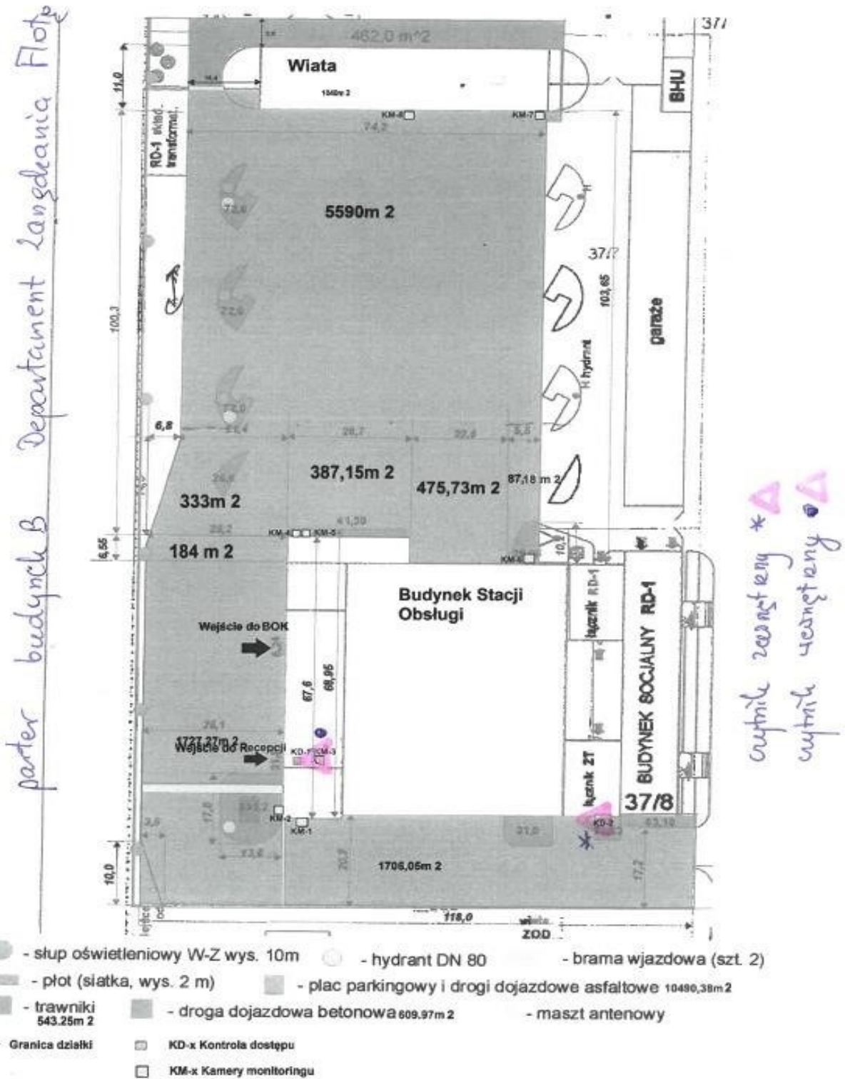
Plan sytuacyjny budynku i działki DZF
